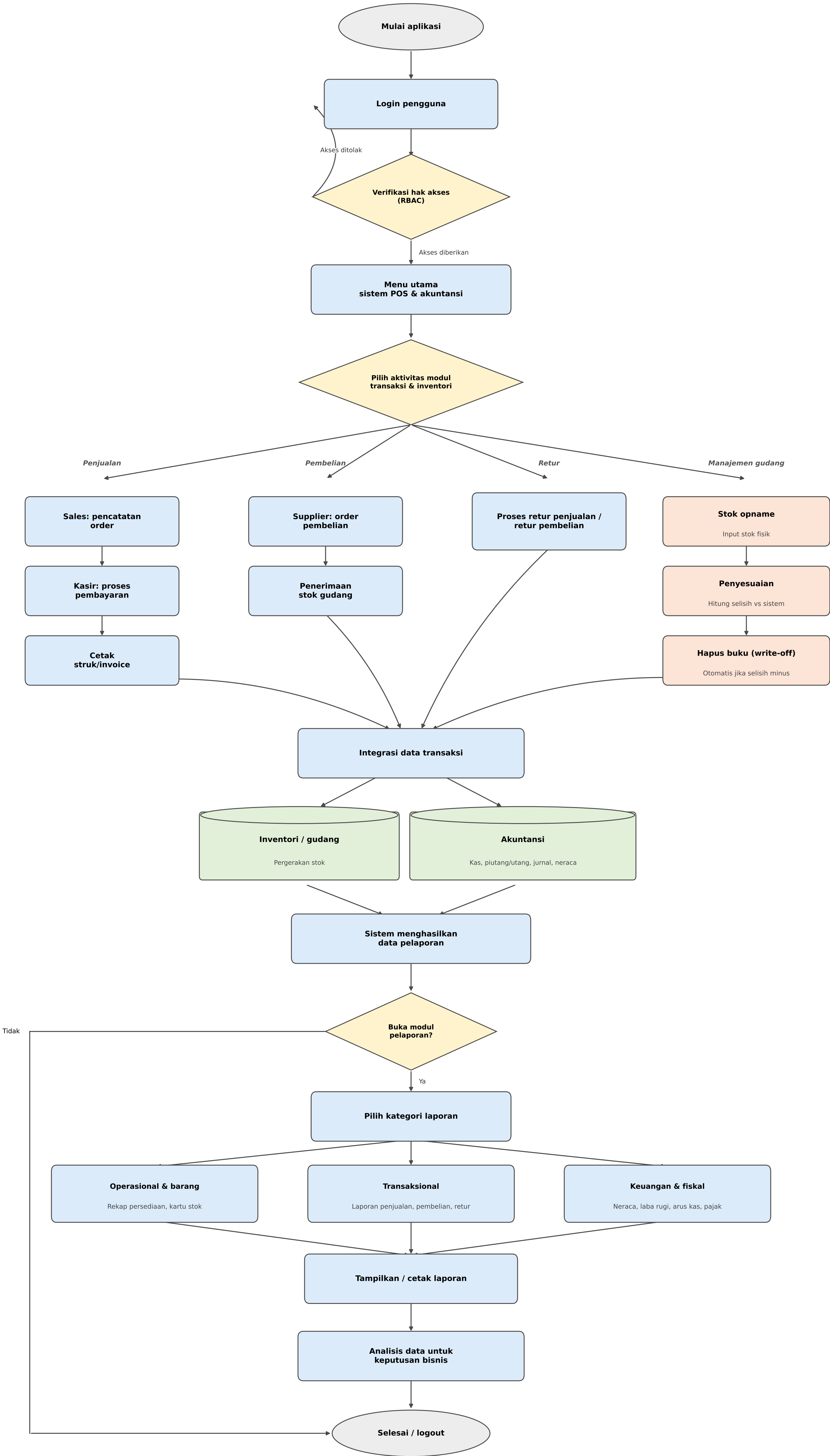
Flowchart Sistem POS & Akuntansi Toko Terintegrasi (versi dikoreksi)
